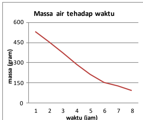
Gambar 13. Grafik massa air yang berkurang di dalam ruang pengering terhadap waktu.
