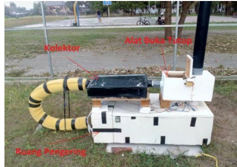
Gambar 7. Rangkaian alat pengujian
