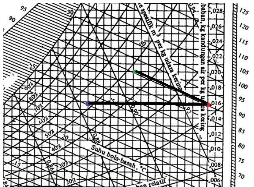
Gambar 10. Hasil pengukuran dengan diagram psikometrik (Visavale, G.L., 2012).
